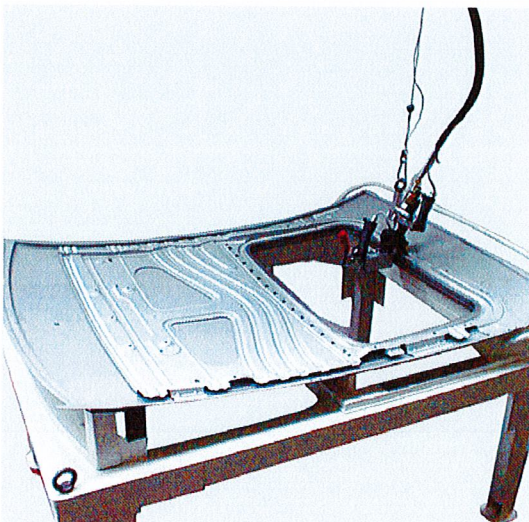
Vorkantwerkzeug FZG-007 Pre-bending tool FZG-007
