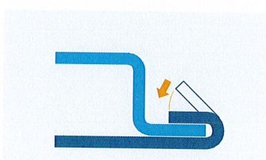
Falzschließen Flachfalz / Seamclosing flat seam
