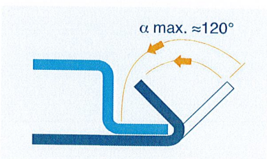
Vorkanten / Pre-bending
