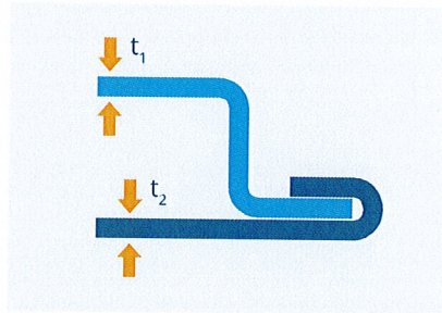
Endstellung Flachfalz End position flat seam
