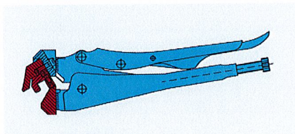
Gripzange mit Falzeinsatz Grip pliers with seamclosing insert
