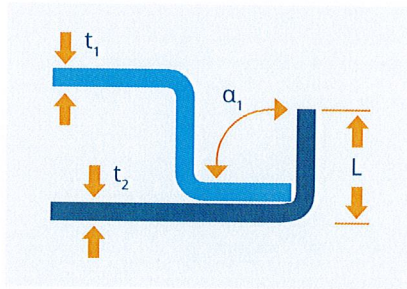
Ausgangsstellung Initial position
