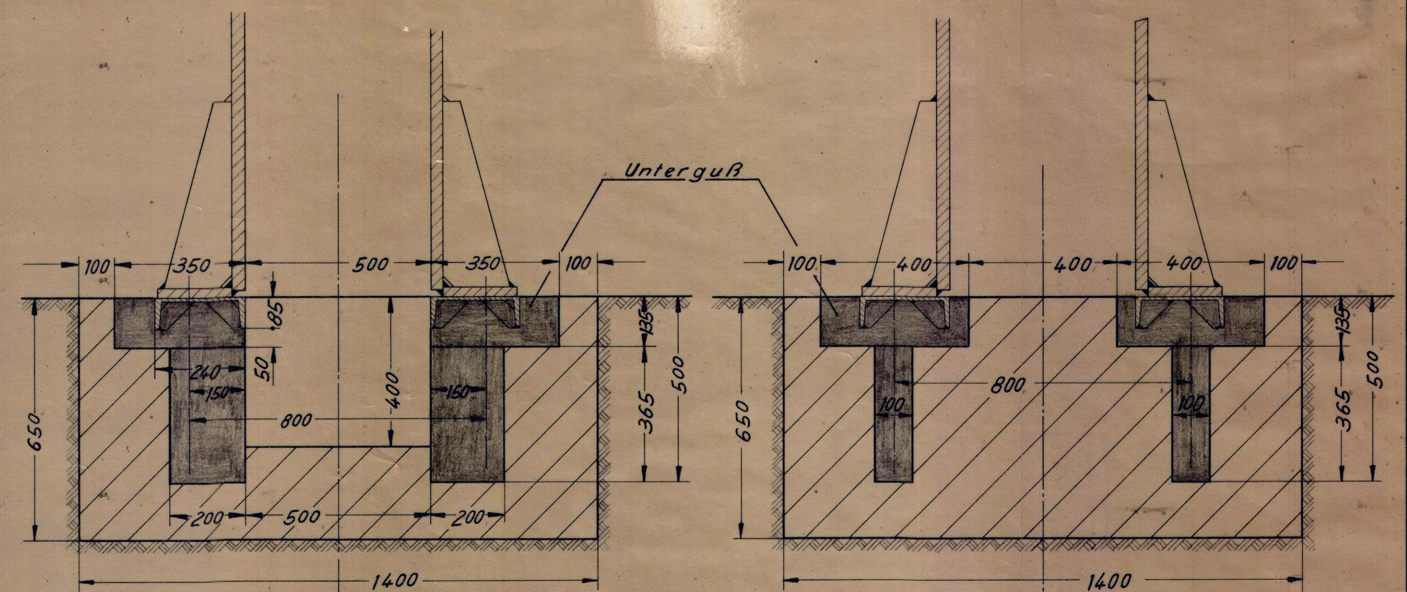
Schnitt: A-A
