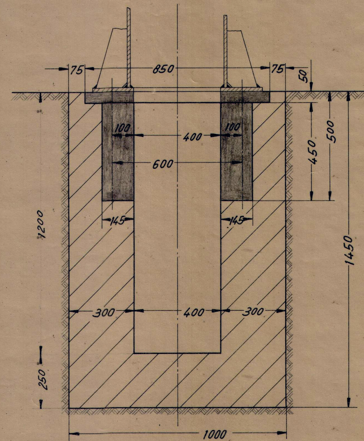
Schnitt: C-C
